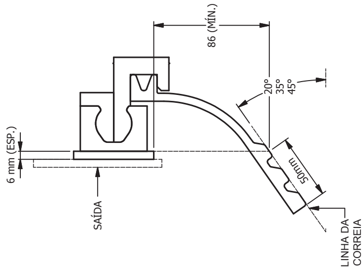
MONTAGEM DA PLACA DE APOIO
