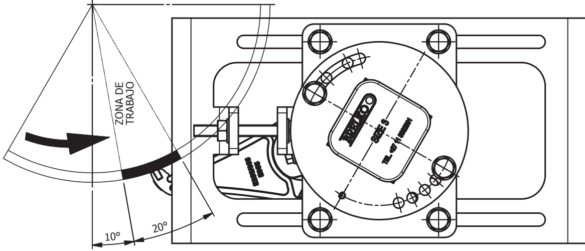
MONTAJE DE TENSOR DE GIRO E955-TT
